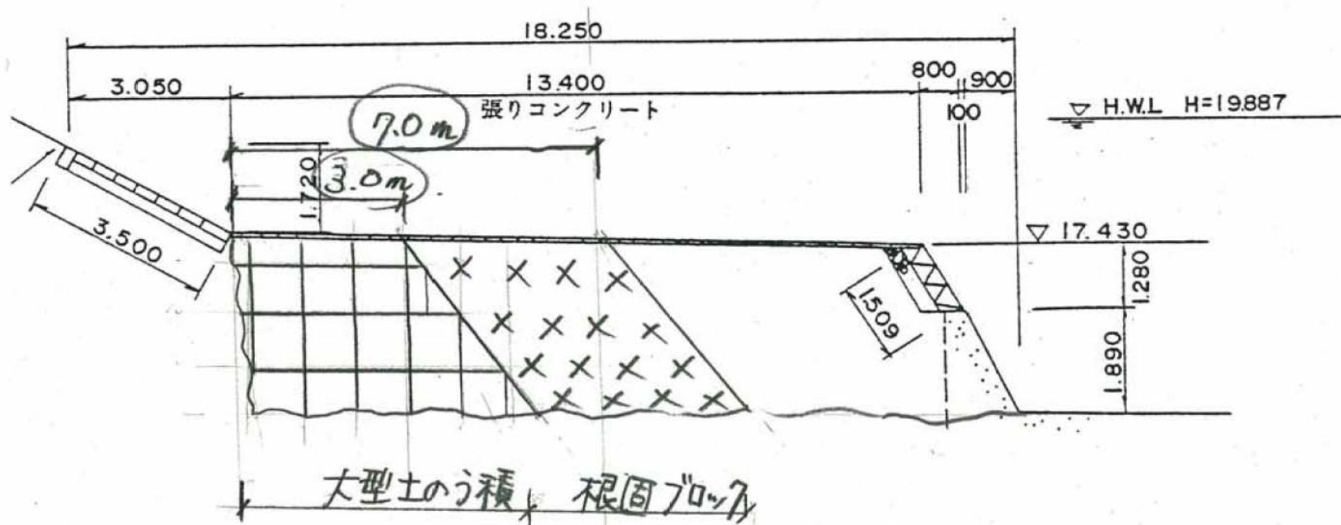
右岸取付護岸横断面図
