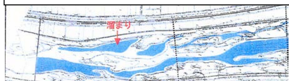
補給前 流量 10.97m 3 /s (平成13年) 河口からの距離 49.40km
