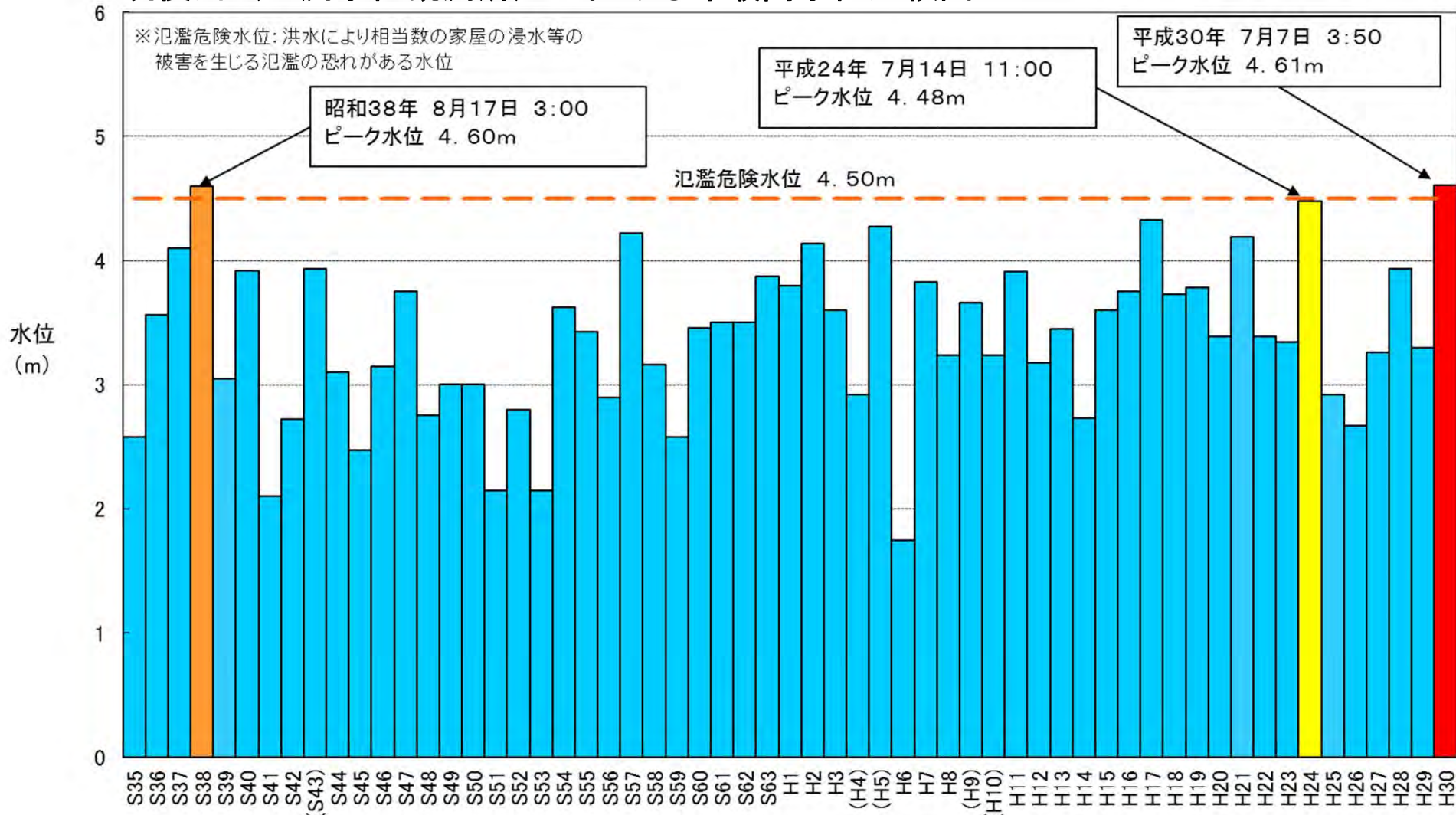
筑後川（小湊水位観測所）における年最高水位比較図
