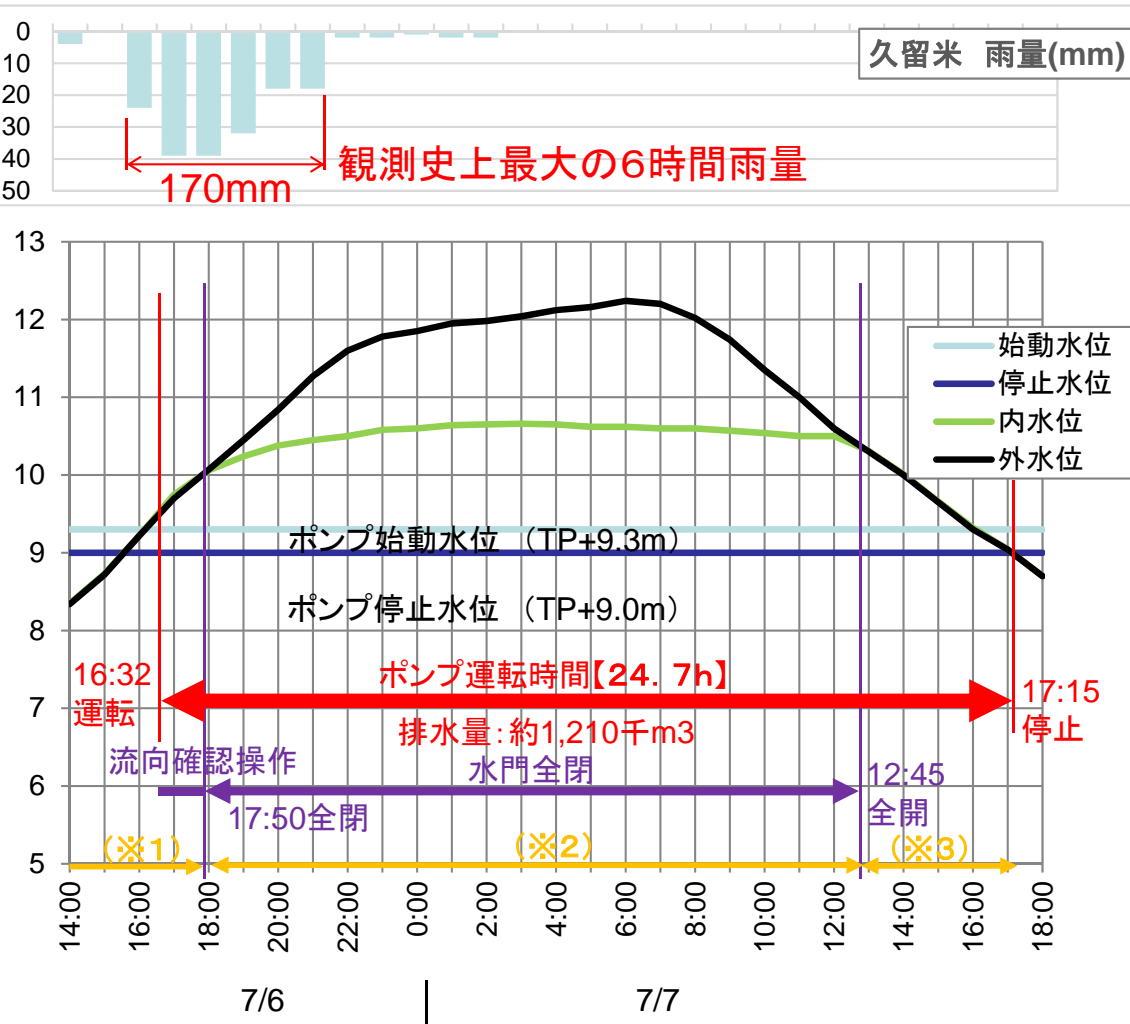
陣屋川排水機場 水位－運転状況
