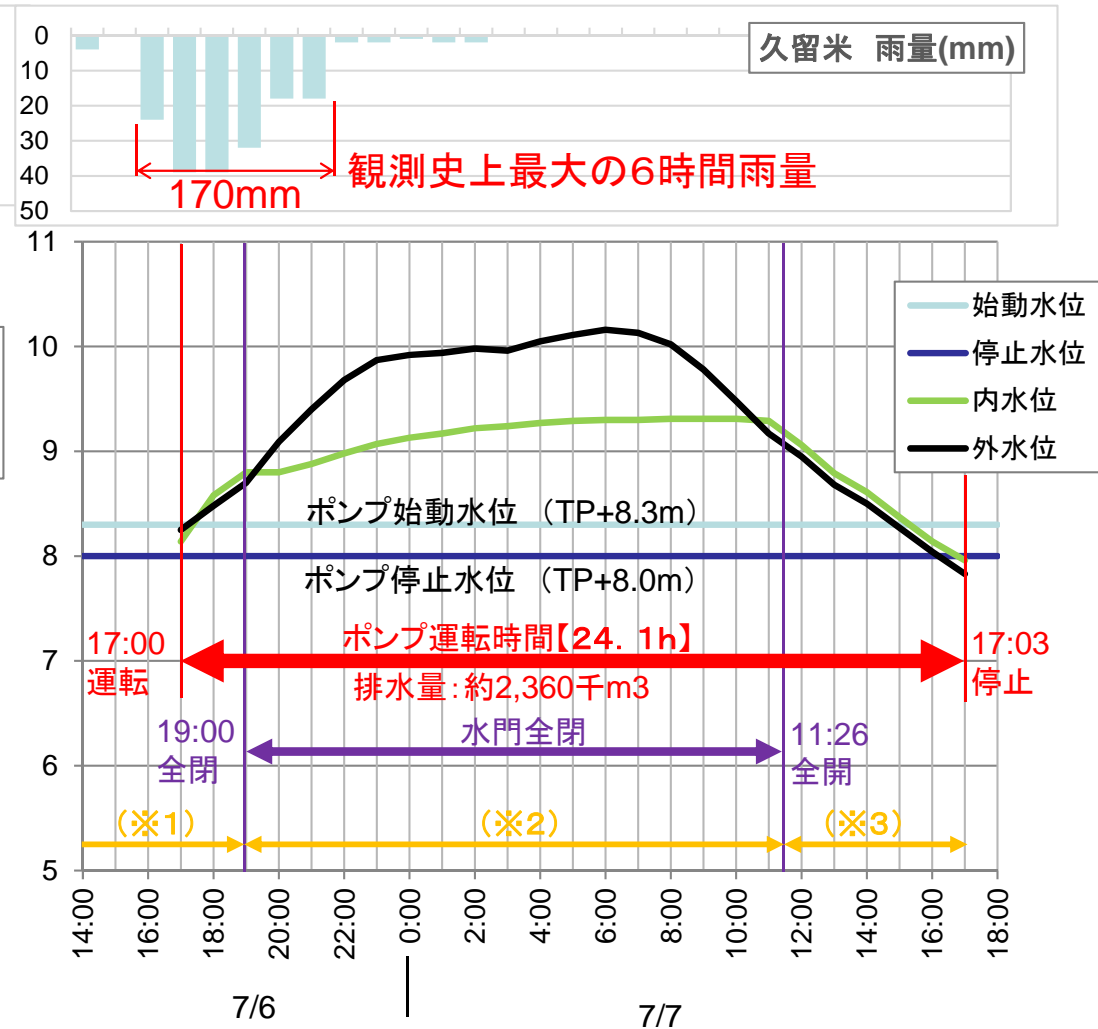
大刀洗排水機場 水位－運転状況
