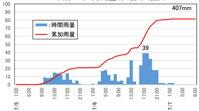
平成30年7月雨量(久留米(国))
