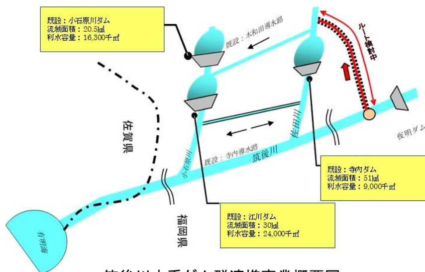
筑後川水系ダム群連携事業概要図
