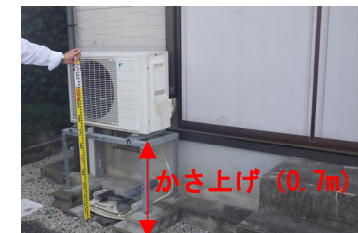
室外機の設置高所化事例
