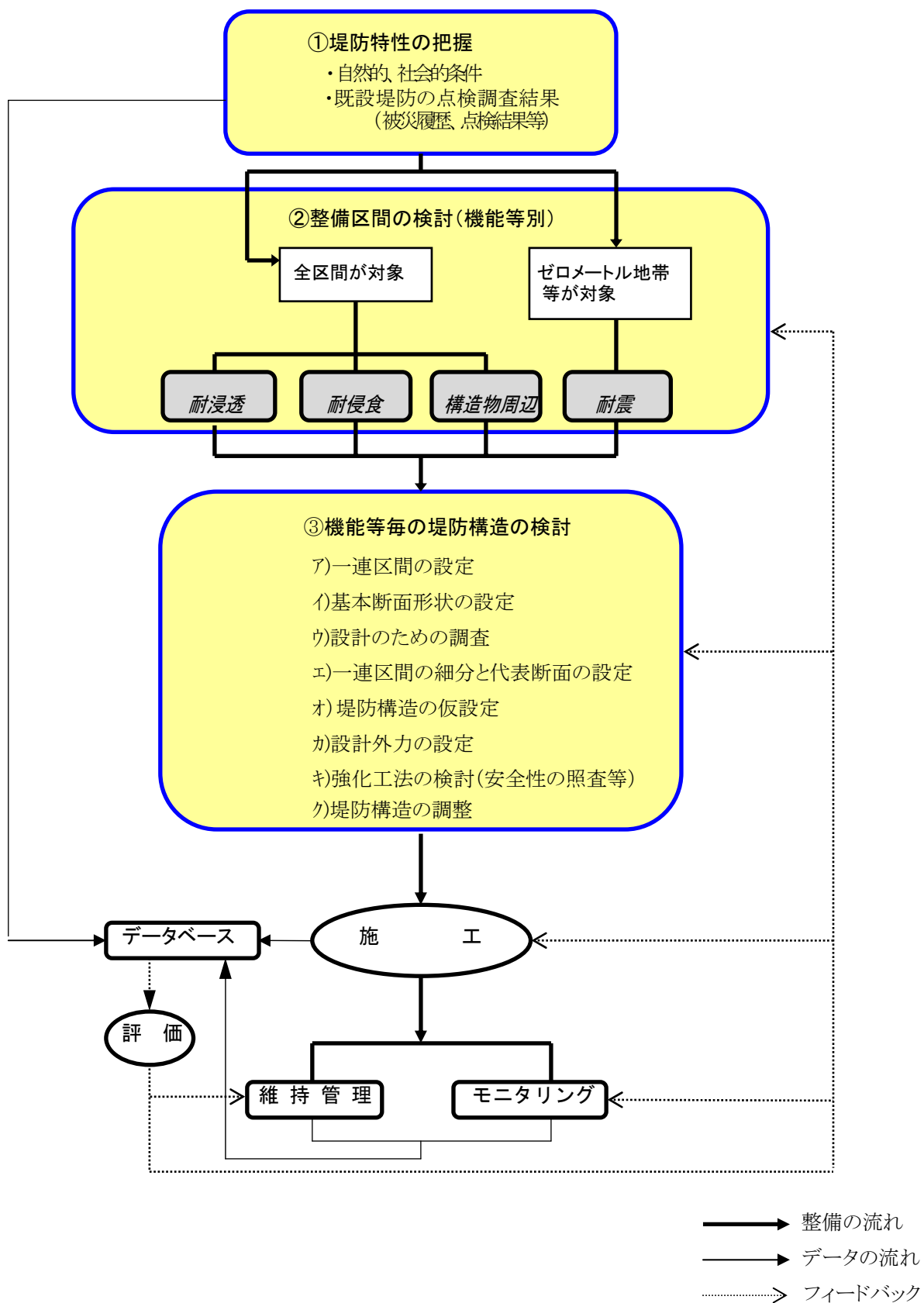
図1 堤防設計の基本的な流れ
