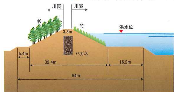
●千栗堤防の断面図（堤防の形）
