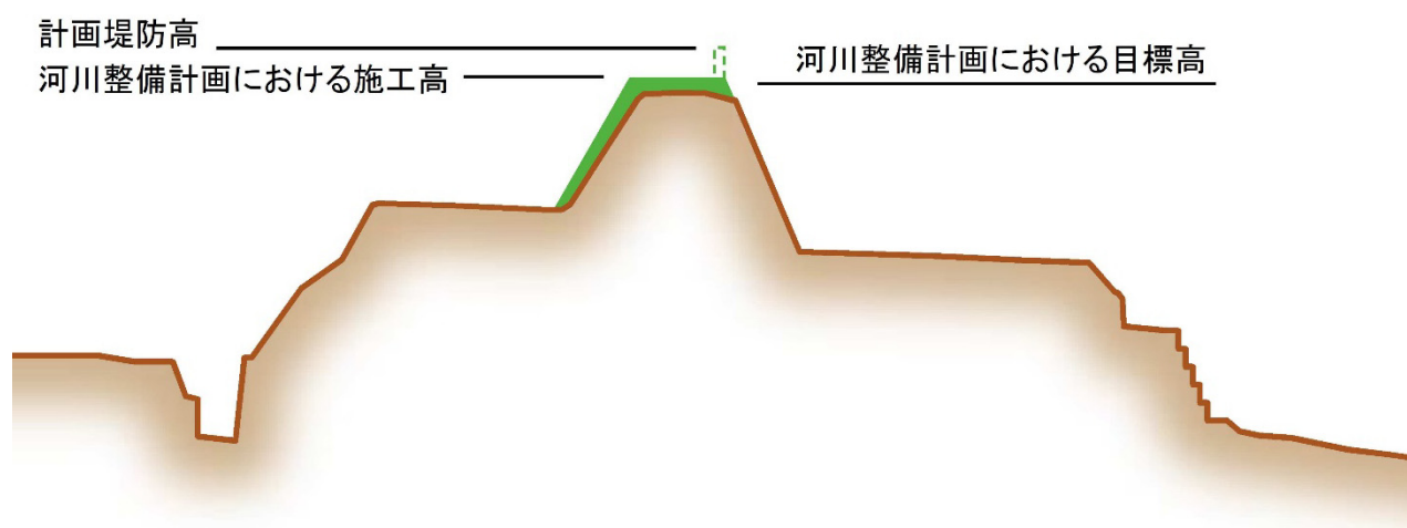
図 4－2－2 0 代表横断面図（川副町大宅間）
