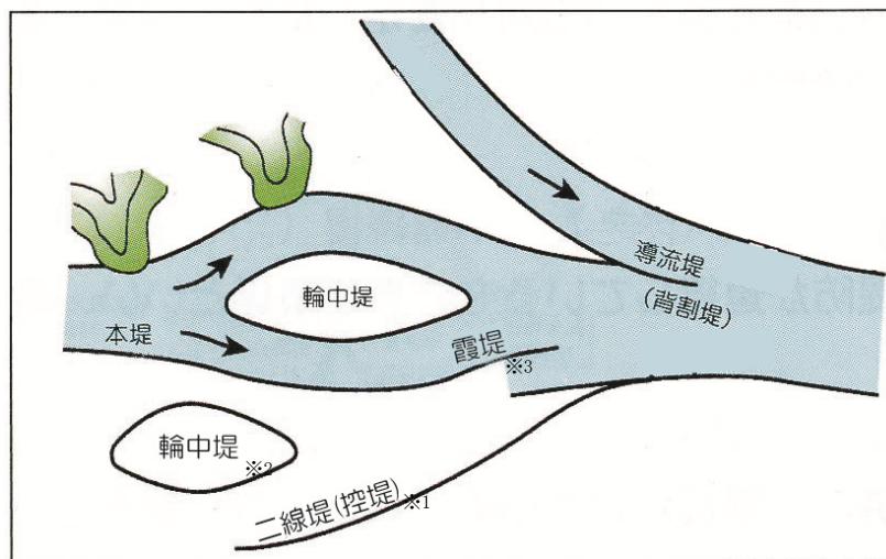
図 4 - 3 - 6 歴史的な治水施設の概要図
