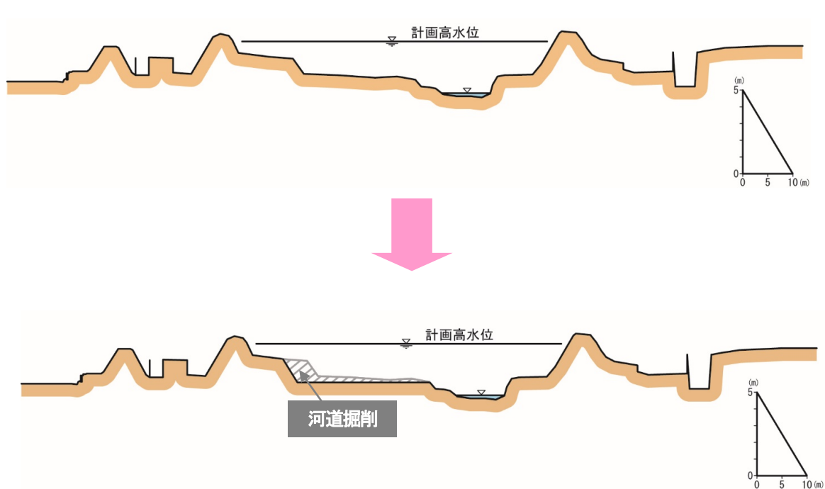
図 4 - 2 - 1 6 代表横断面図（左岸、右岸：朝倉市屋永）
