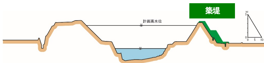
図 4-2-9 代表横断面図（右岸：久留米市大善寺町中津）
