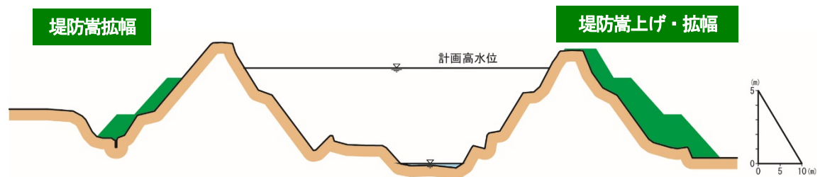
図 4-2-11 代表横断面図（左岸：鳥栖市真木町、右岸：鳥栖市下野町）
