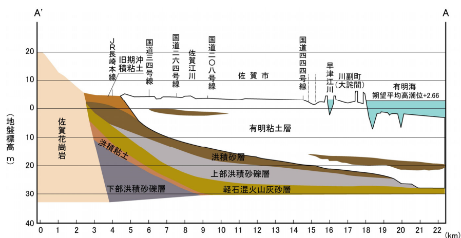
図 1-1-4 佐賀平野の地質横断面図 (A'-A 断面)
