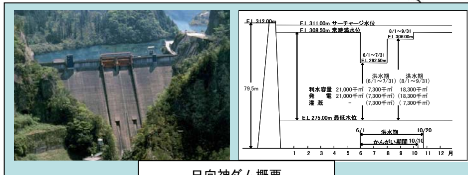
日向神ダム概要
