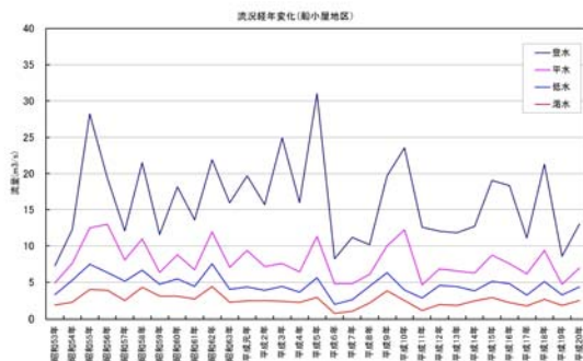
図 3.2.5 矢部川水系の流況
