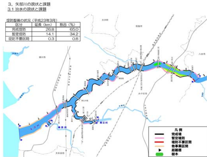
図 3.1.1 堤防整備状況図
