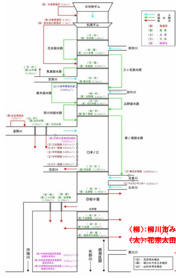
図 3.2.2 矢部川水系の主な水利用の現況模式図 ※干出量、下名競渡は水利種における名称です。本計画では、干出量を大和量、下名競渡を名競渡と表記しています
