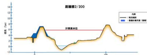
図 5.2.6 堤防整備の概要図(飯江川左岸 2/200 付近)
