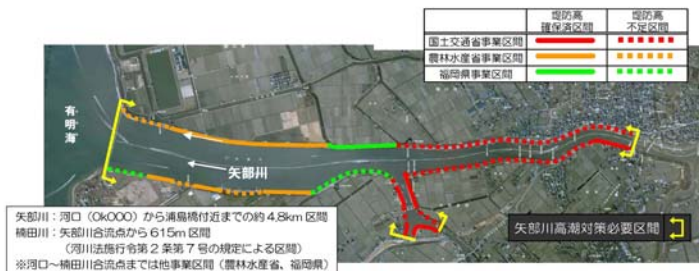
図 3.1.3 矢部川高潮対策必要区間
