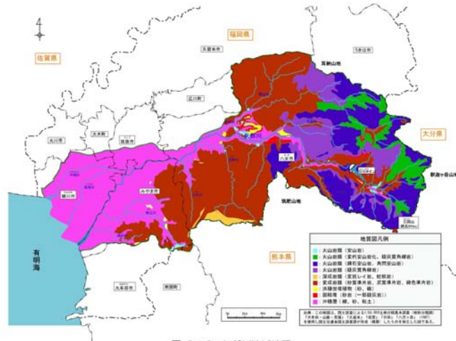
図 2.1.6 矢部川流域地質
