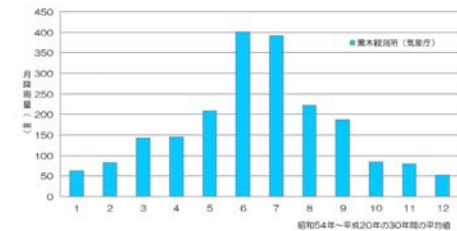
図 2.1.10 主要地点の月別降水量
