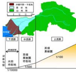
図 2.1.5 矢部川地形模式図
