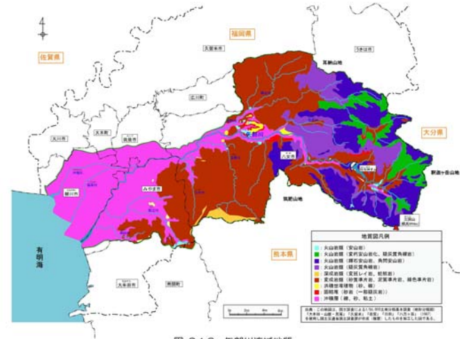
図 2.1.6 矢部川流域地質
