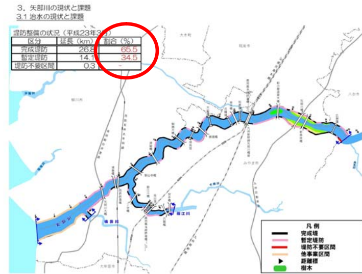
図 3.1.1 堤防整備状況図
