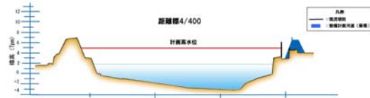
図 5.2.5 堤防整備の概要図(矢部川右岸 4/400 付近)
