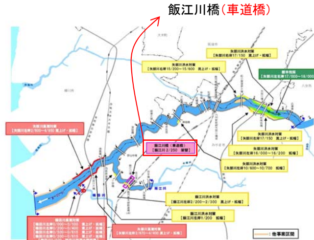
図 5.2.2 河川整備位置図
