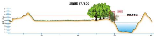
図 5.2.7 樹木伐採の概要図(矢部川 17/600 付近)
