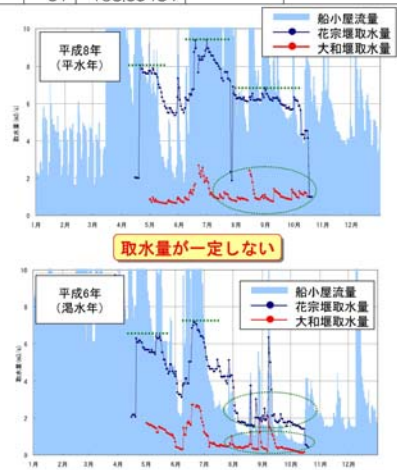
図 3.2.4 矢部川水系の取水実態
