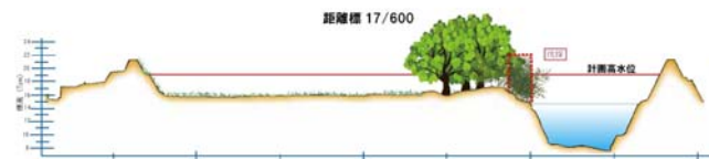
図 5.2.6 樹木伐採の概要図(矢部川 17/600 付近)
