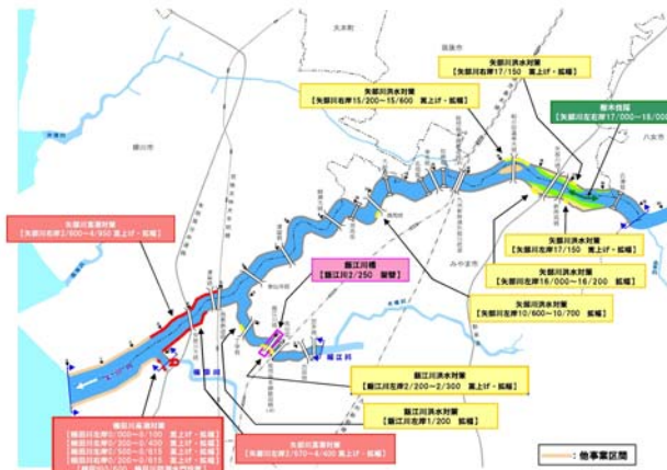
図 5.2.3 河川整備位置図
