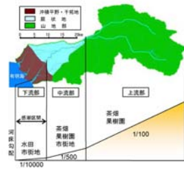
図 2.1.5 矢部川地形模式図
