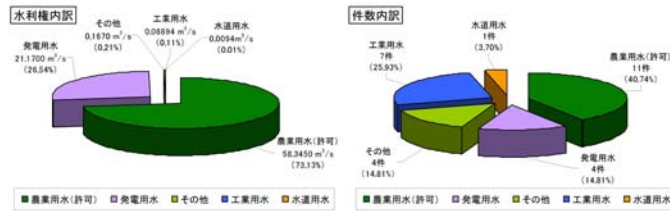
図 3.2.3 矢部川水系における水利権
