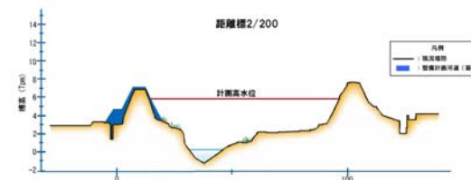
図 5.2.5 堤防整備の概要図(飯江川左岸 2/200 付近)
