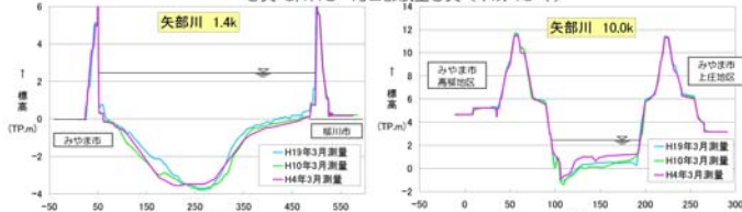
図 3.1.9 横断面重ね合わせ図 (矢部川河口より 1k400 地点)
