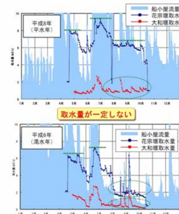
図 3.2.4 矢部川水系の取水実態
