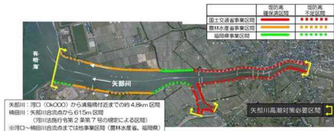
図 3.1.3 矢部川高潮対策必要区間
