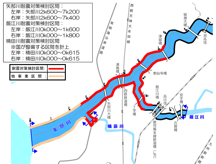
図 3.1.6 矢部川水系堤防耐震対策検討区間-国管理区間-
