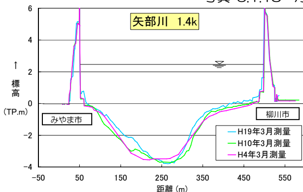
図 3.1.9 横断面重ね合わせ図 (矢部川河口より 1k400 地点)
