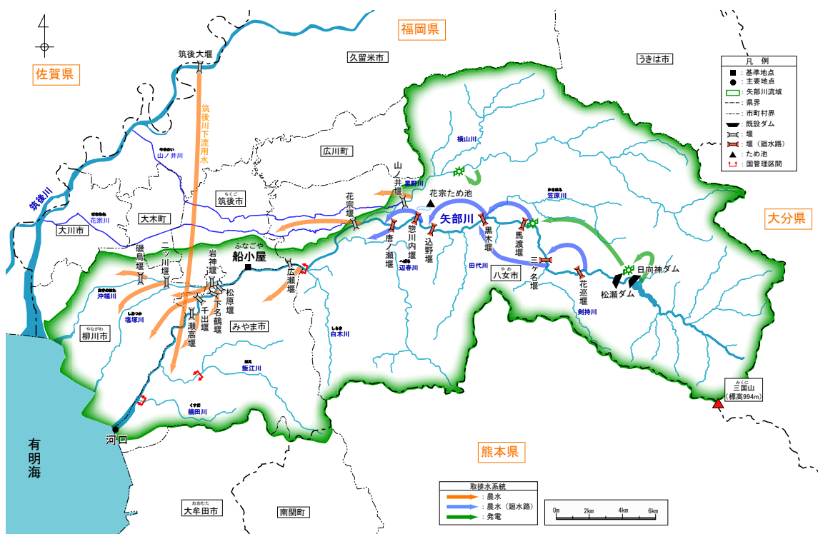
図 3.2.1 矢部川水系取水排水系統と主な利水施設
