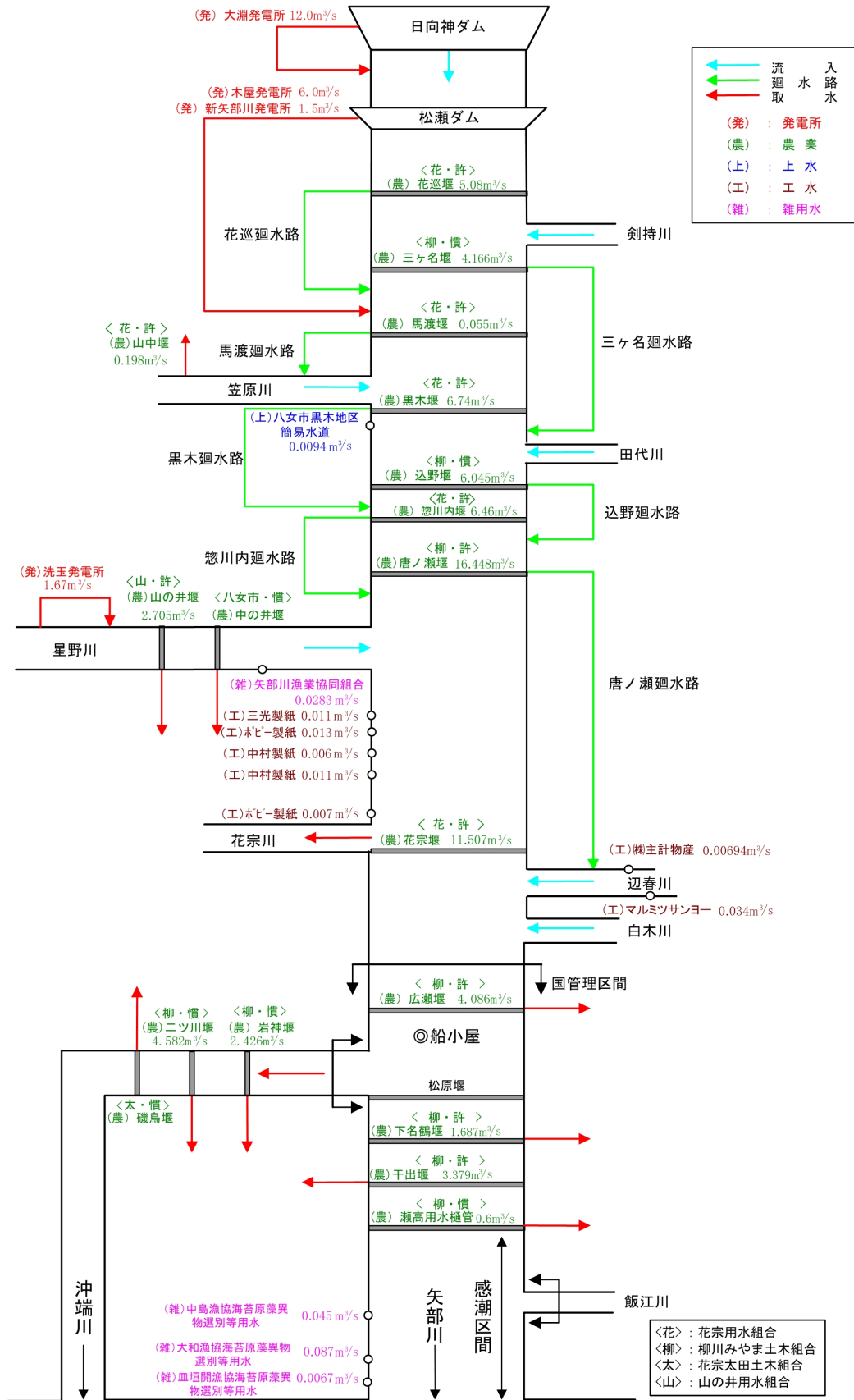
図 3.2.2 矢部川水系の主な水利用の現況模式図
