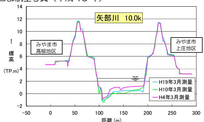
図 3.1.10 横断面重ね合わせ図 (矢部川河口より 10k000 地点)
