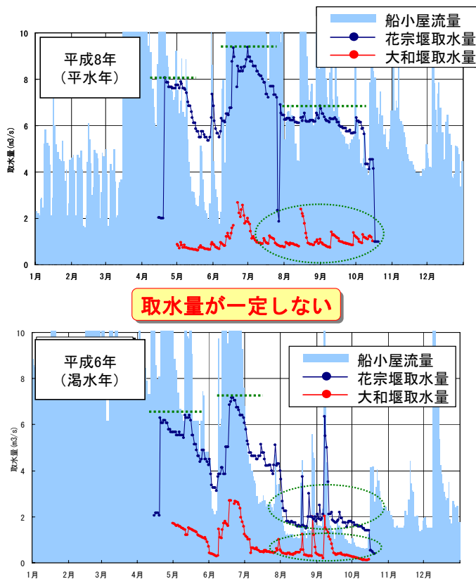
図 3.2.4 矢部川水系の取水実態
