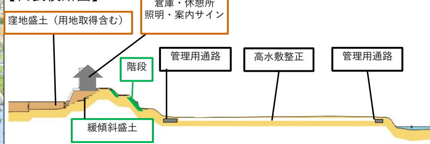
【代表横断面図】
