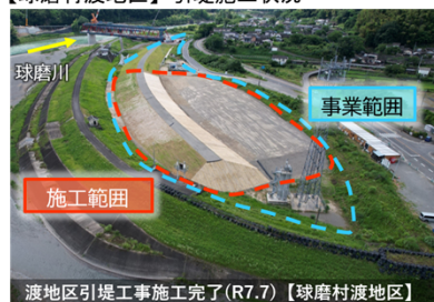
【球磨村渡地区】引堤施工状況
