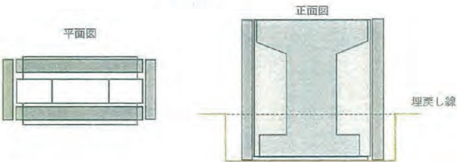
「足場組立図」
