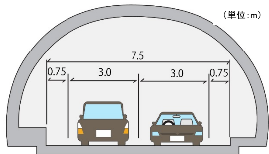
【トンネル部】
