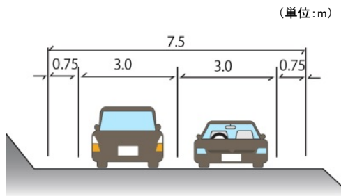
【一般部】
