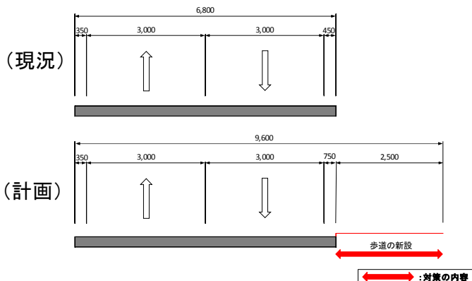
【横断図】
