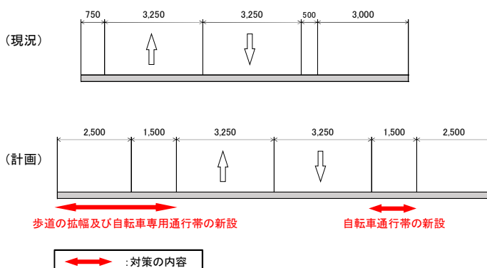
【横断図】
