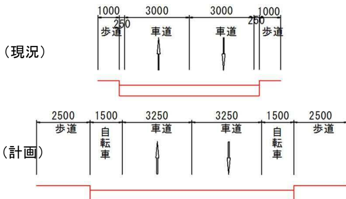
【横断図】
