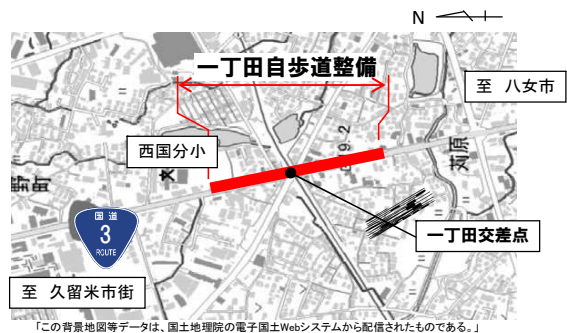
【位置平面図】
