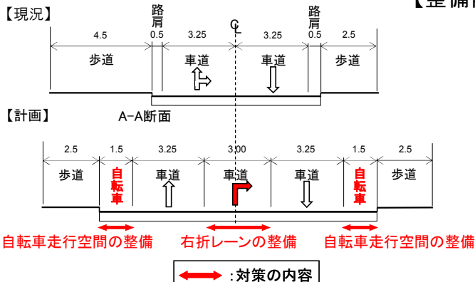
【横断面】
