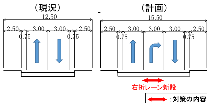
【横断図】
