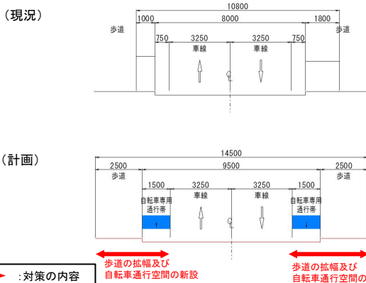
【横断面図】
