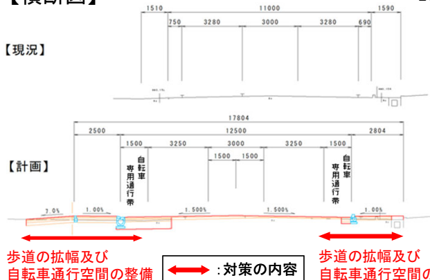
【横断図】
