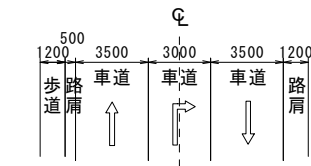
【横断面図】
