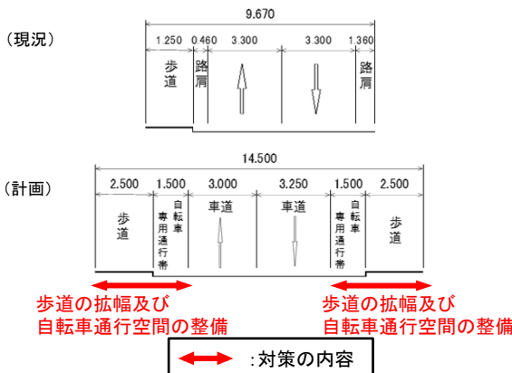
【横断図】
