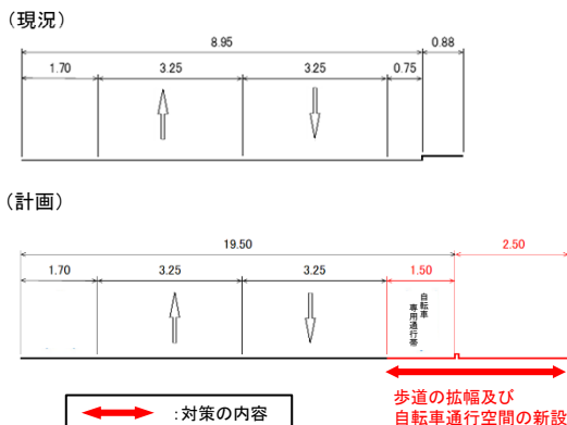
【横断図】
