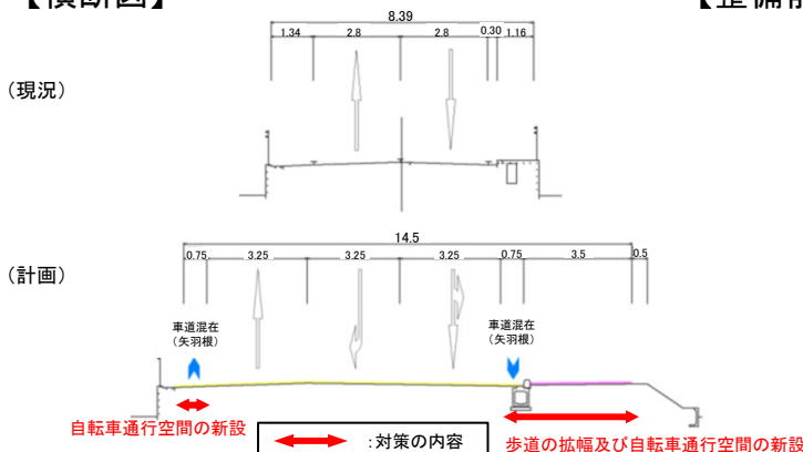
【横断面図】
