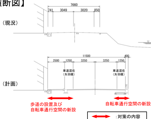
【横断図】
