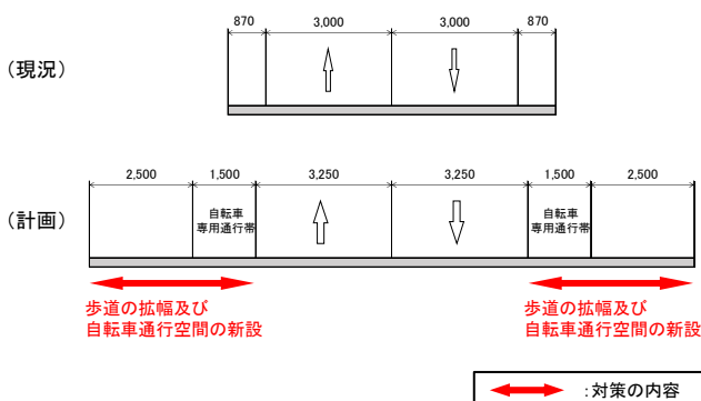
【横断図】
