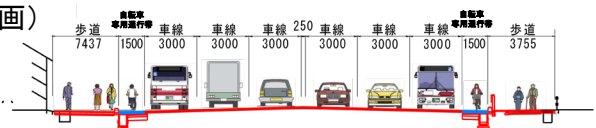
歩道の拡幅及び自転車通行空間の新設 : 対策の内容 歩道の拡幅及び自転車通行空間の新設
