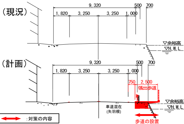
【横断面図】
