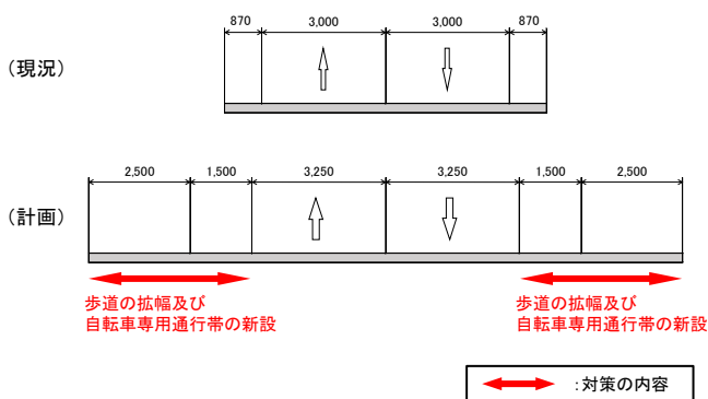
【横断図】
