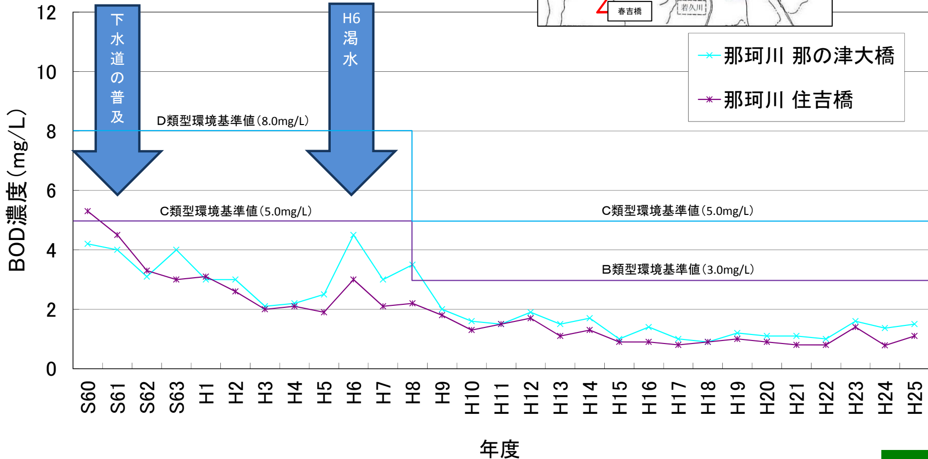
■那珂川水系BOD濃度(年平均)経年変化
