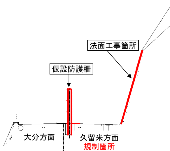
工事区間概略横断面図
