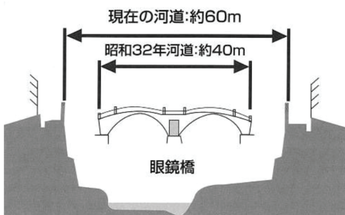
眼鏡橋地点の川幅の拡幅
