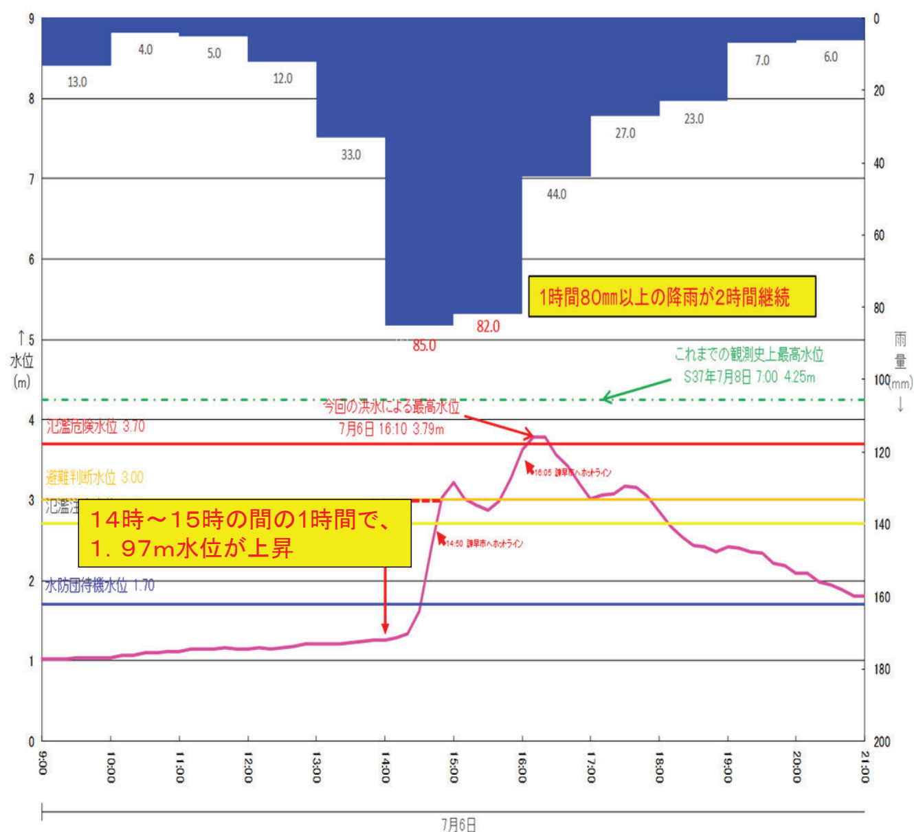
令和2年7月6日出水 裏山水位観測所—小野雨量観測所
