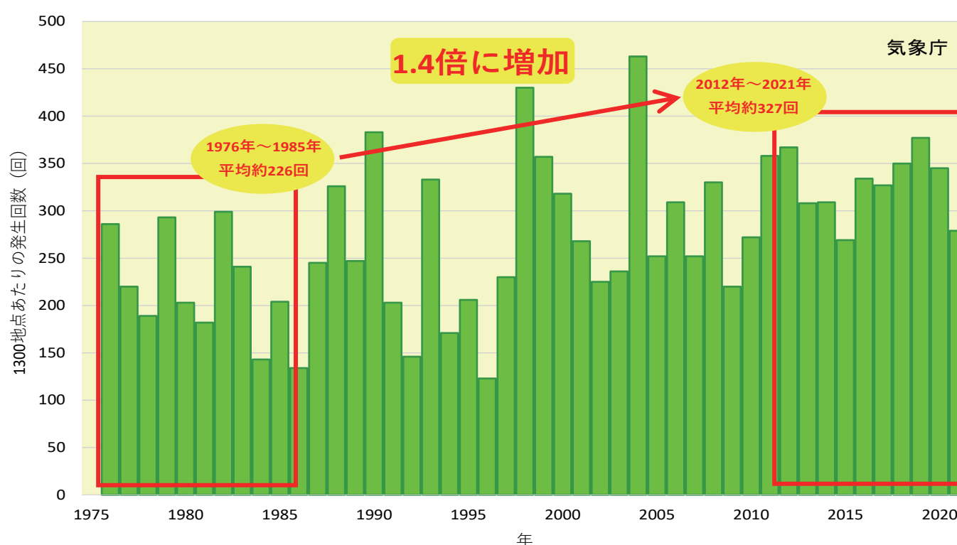
図 全国の1時間降水量50mm以上の年間発生回数の経年変化（1976年～2021年）
