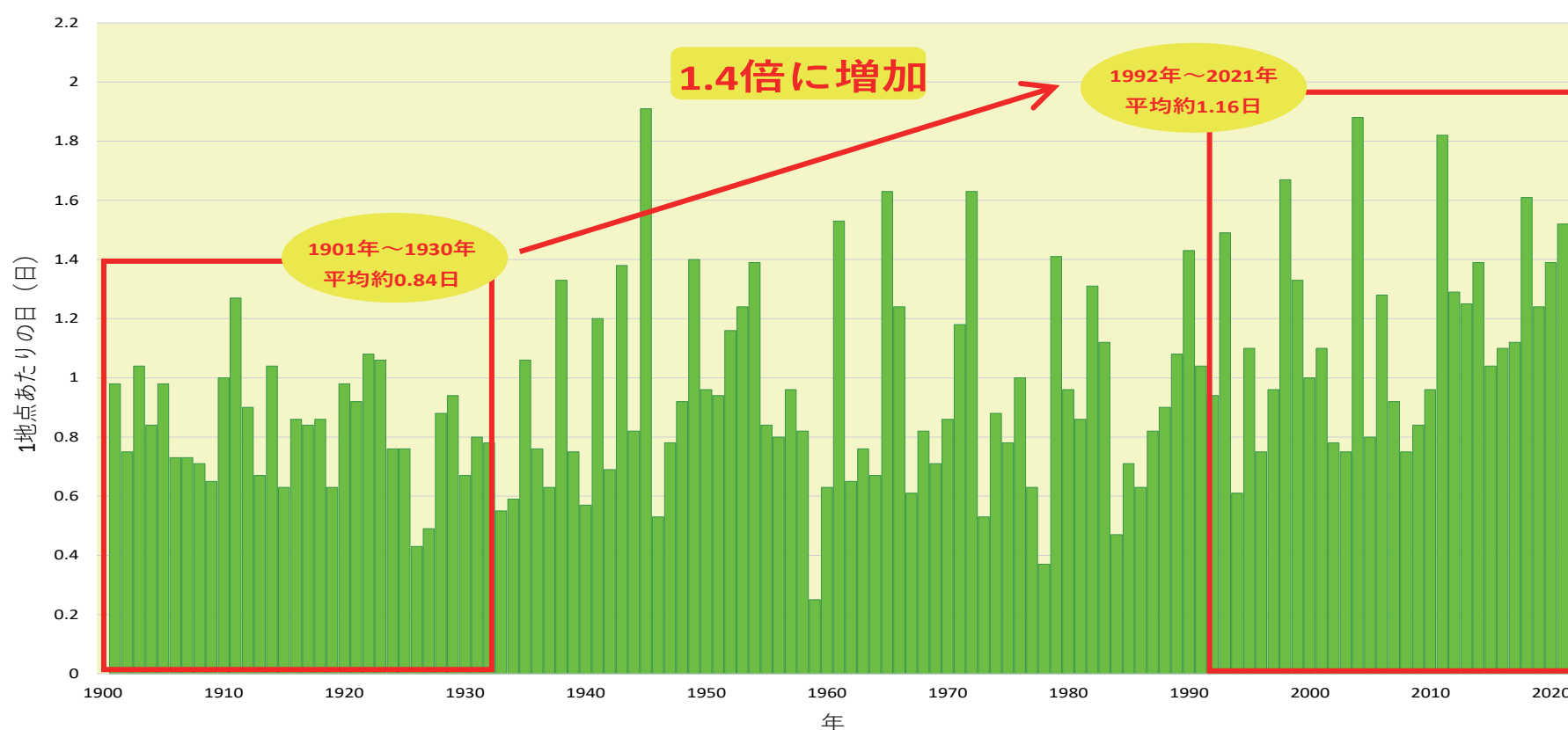
図 全国の日降水量100mm以上の年間日数の経年変化（1901年～2021年）
