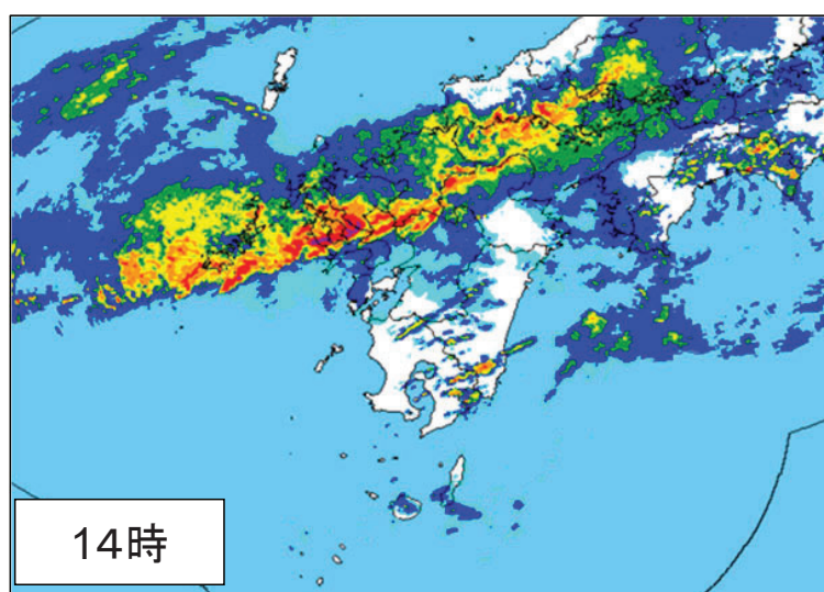
令和2年7月6日の雨雲の動き
