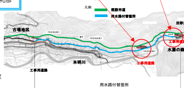
全体平面図
