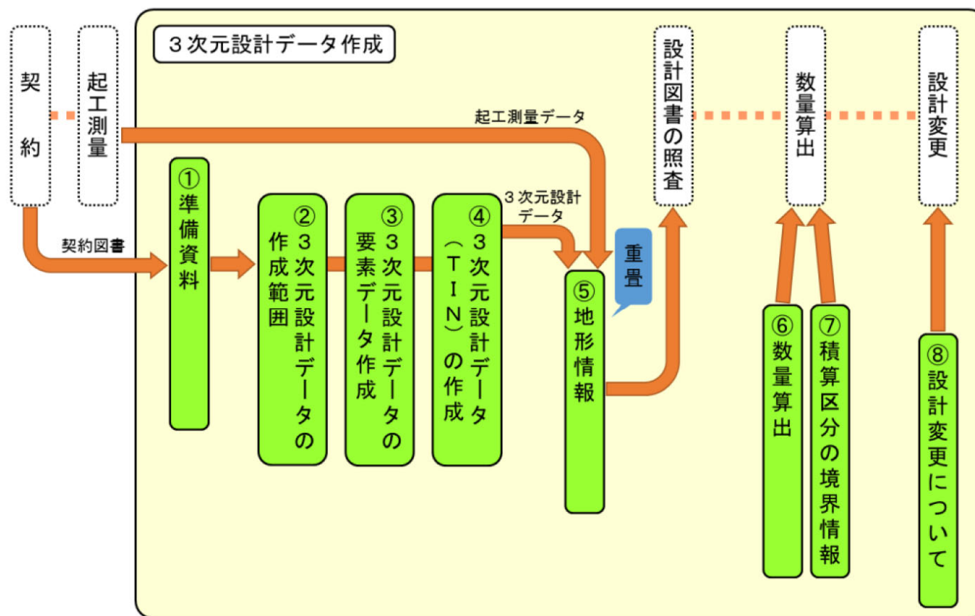
3次元設計データ作成の流れ
