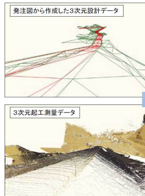
起工測量結果と3次元設計データ
