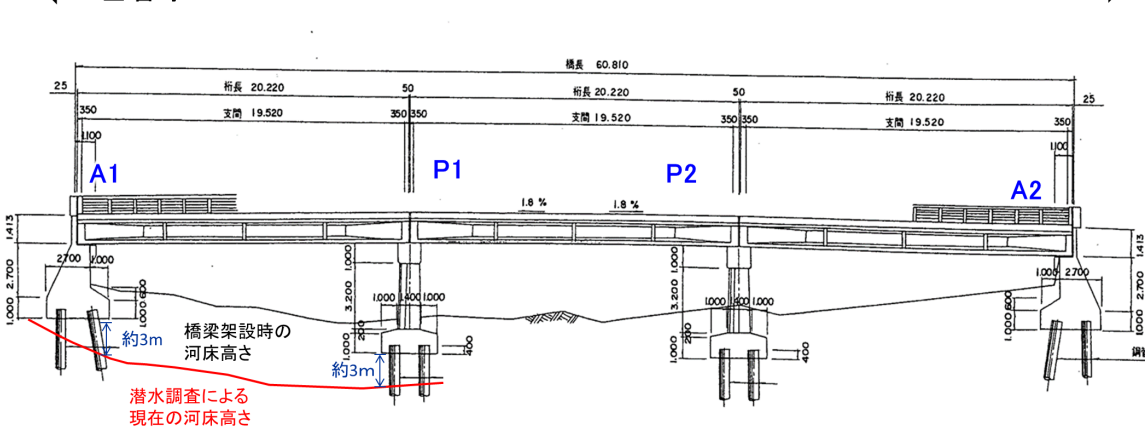
側面図
