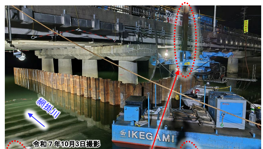
▼桁下に設置している短い鋼矢板
