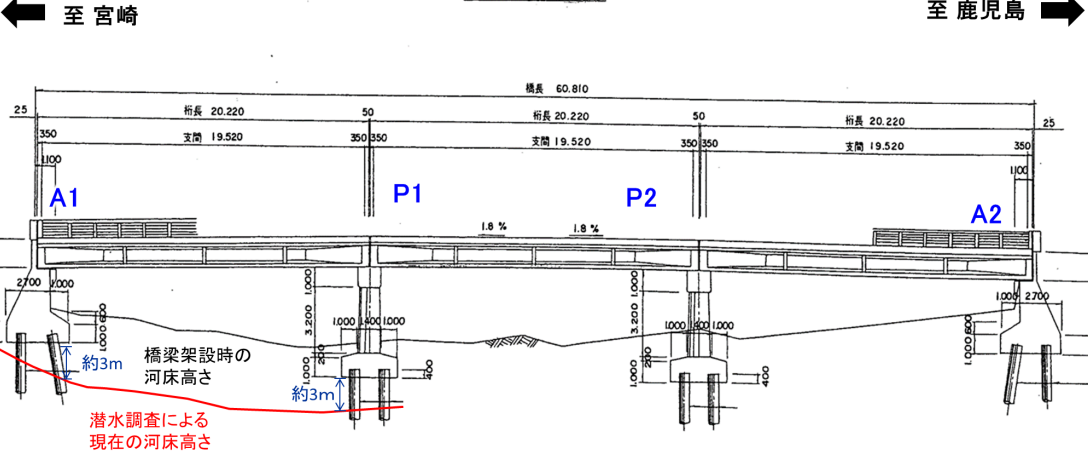
側面図
