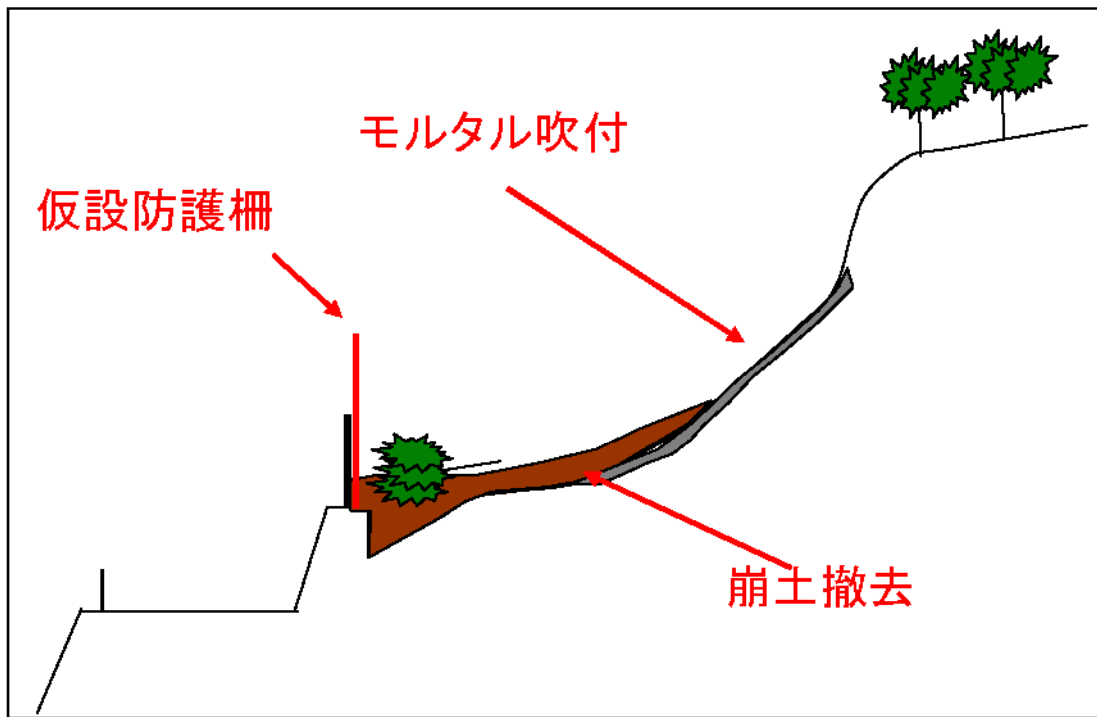
横断図
