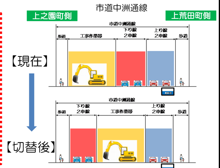
◇横断図
