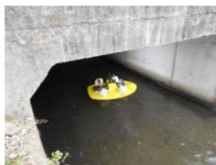
水上ドローンによる損傷把握
