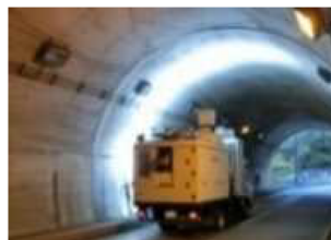
レーザースキャンによる変状把握
