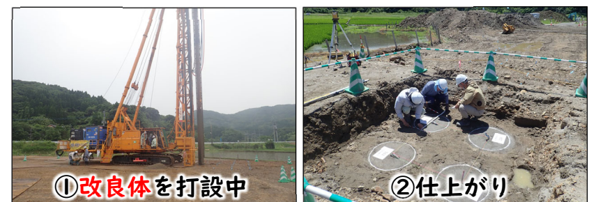
サンドコンパクションパイル工法
