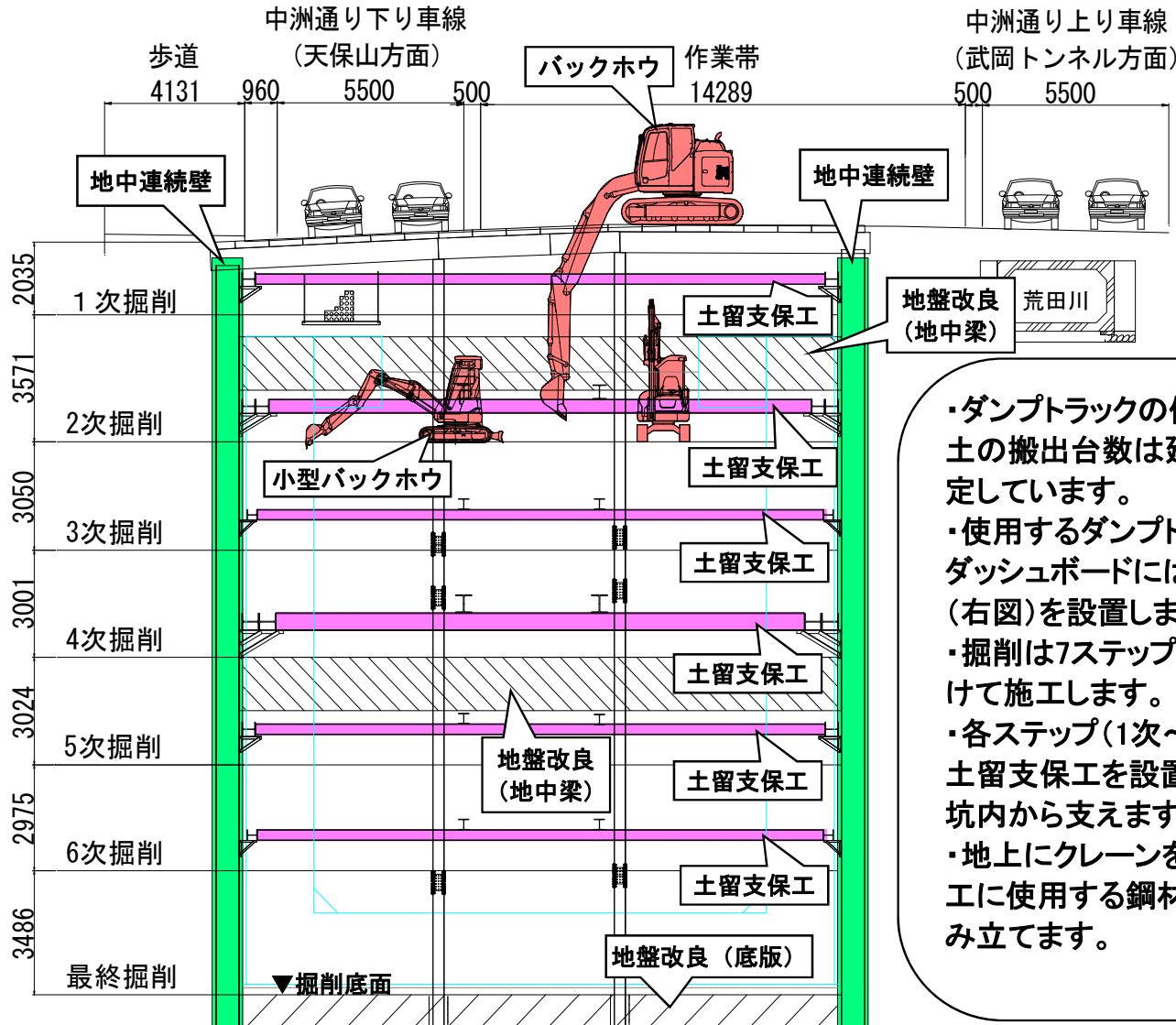
掘削工、土留支保工 断面図
