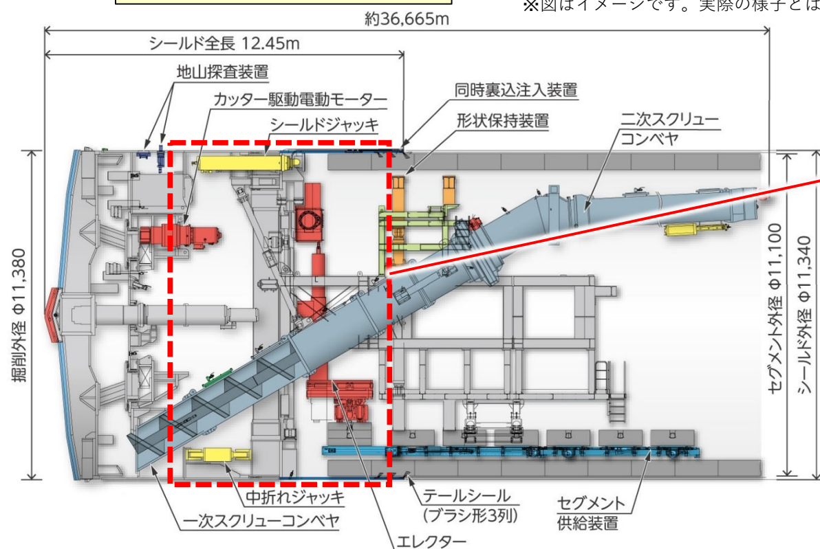
シールドマシンの側面断面図
