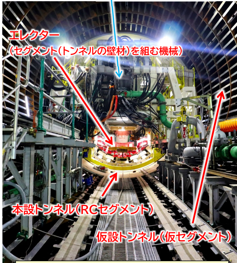
トンネル内からシールドマシン後方を見た状況
