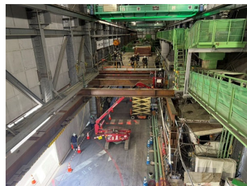
作業床 (2F部分) の撤去
