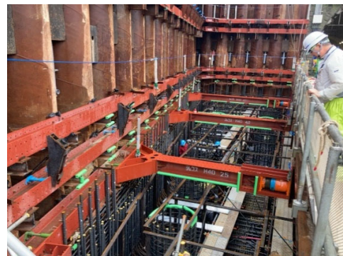
鉄筋架台設置状況
