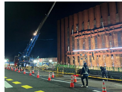
鉄筋組立作業状況 (夜間)
