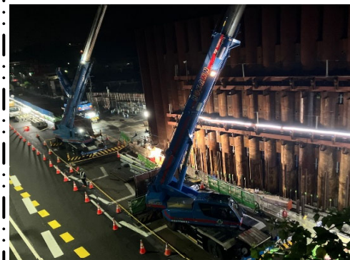
鉄筋架台設置状況（夜間）
