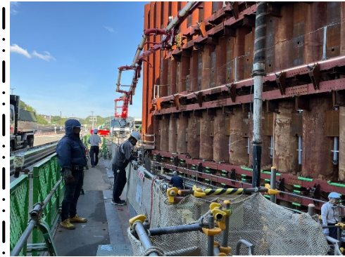
コンクリート打設作業状況
